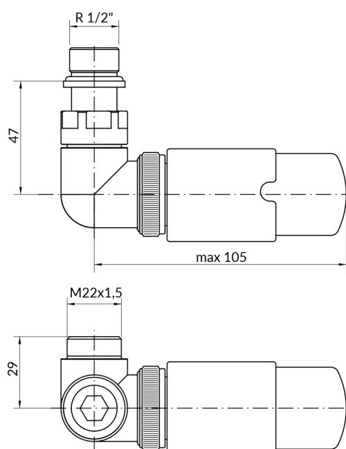
Dreiachsiges Regelventil
