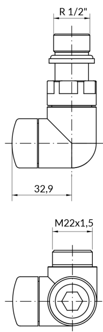
Dreiachsiges Absperrventil
