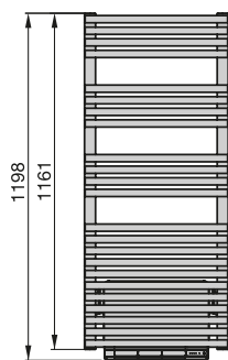
Vorderansicht, LF(C)-120
