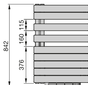
Vorderansicht, ROFR-090
