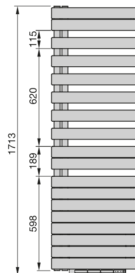
Vorderansicht, ROFR-180
