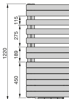
Vorderansicht, ROFR-130
