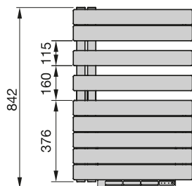
Vorderansicht, ROFR-090
