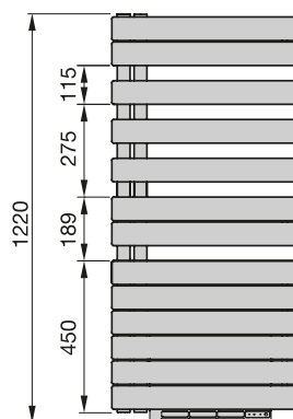
Vorderansicht, ROFR-130
