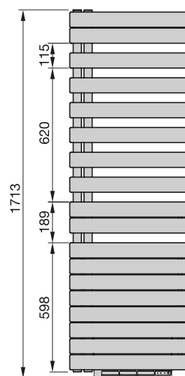
Vorderansicht, ROFR-180
