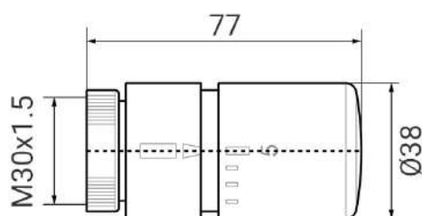
Abmessungen thermostatkopf
