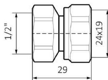
Abmessungen adapter Stahl
