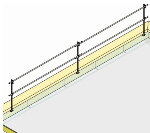
2 – Konfiguration mit 2 Stängen
