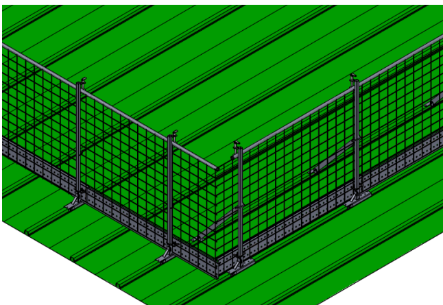
1 – Konfiguration mit Netz und 1 Stange
