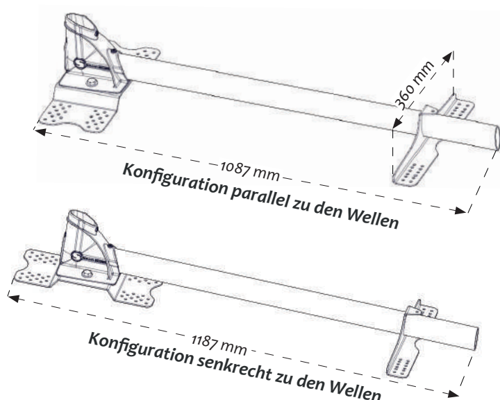
Art.Nr: 100543 Stützstrebe
