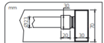
Dimensioni corpo radiatore
