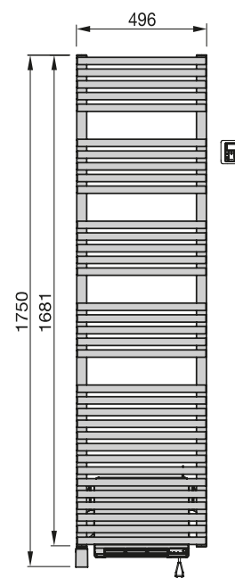
Vista frontale LFE-170-050
