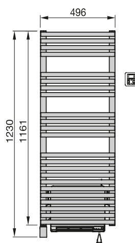
Vista frontale LFE(C)-120-050
