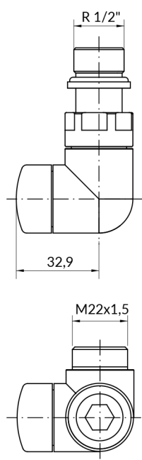
Valvola di interruzione triassiale
