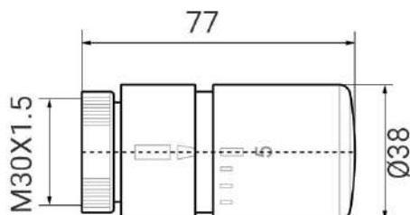
Tête thermostatique
