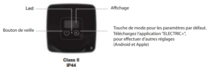
Chronothermostat avec gestion Bluetooth par smartphone
